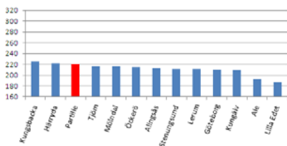
Genomsnittligt meritvärde
